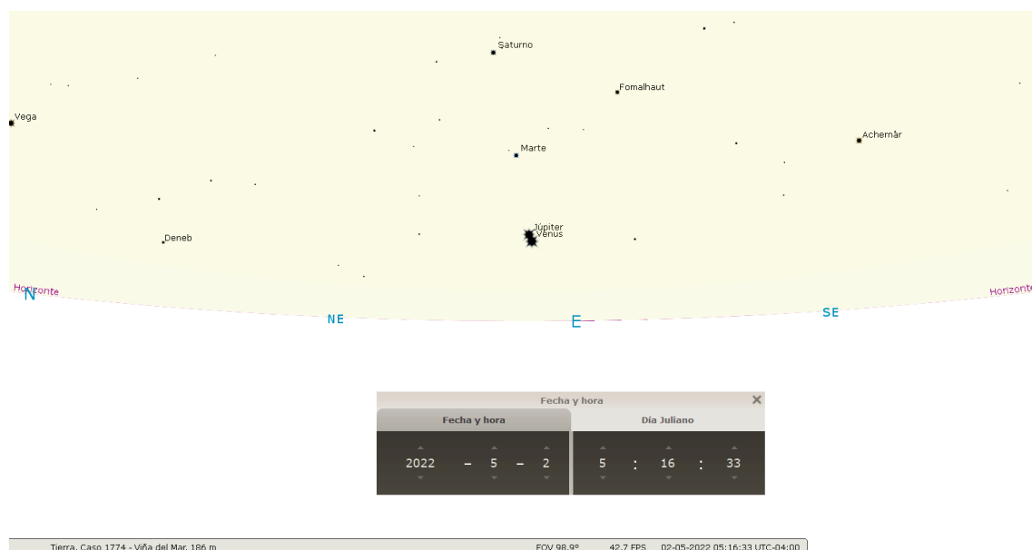
Figura 3. Horizonte astronómico visible por la usuaria al momento de captar la imagen.
